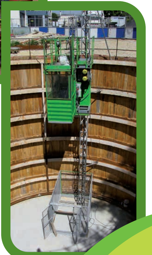
Fin des opérations de préparation de la fosse accédant aux cuves d'entreposage.
